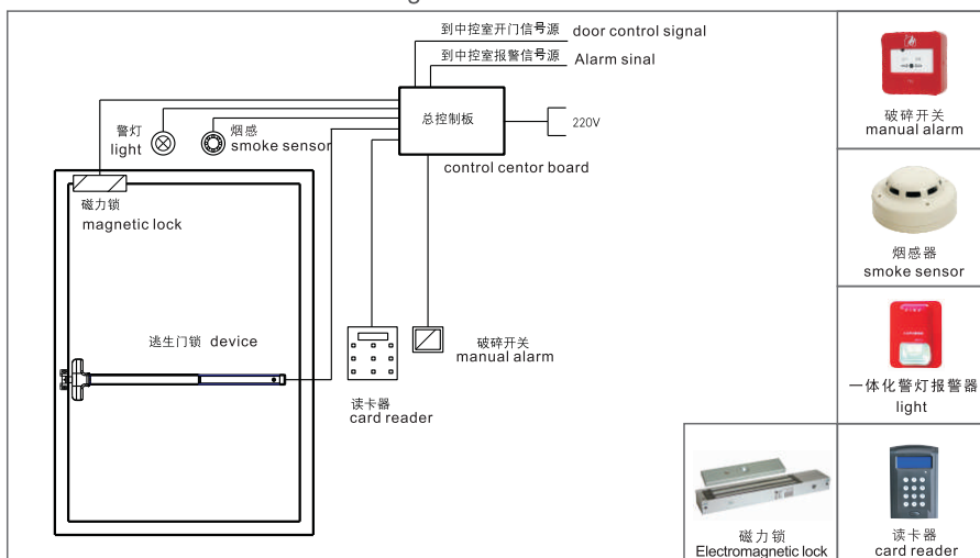
线路安装示意图 Installation Diagram
