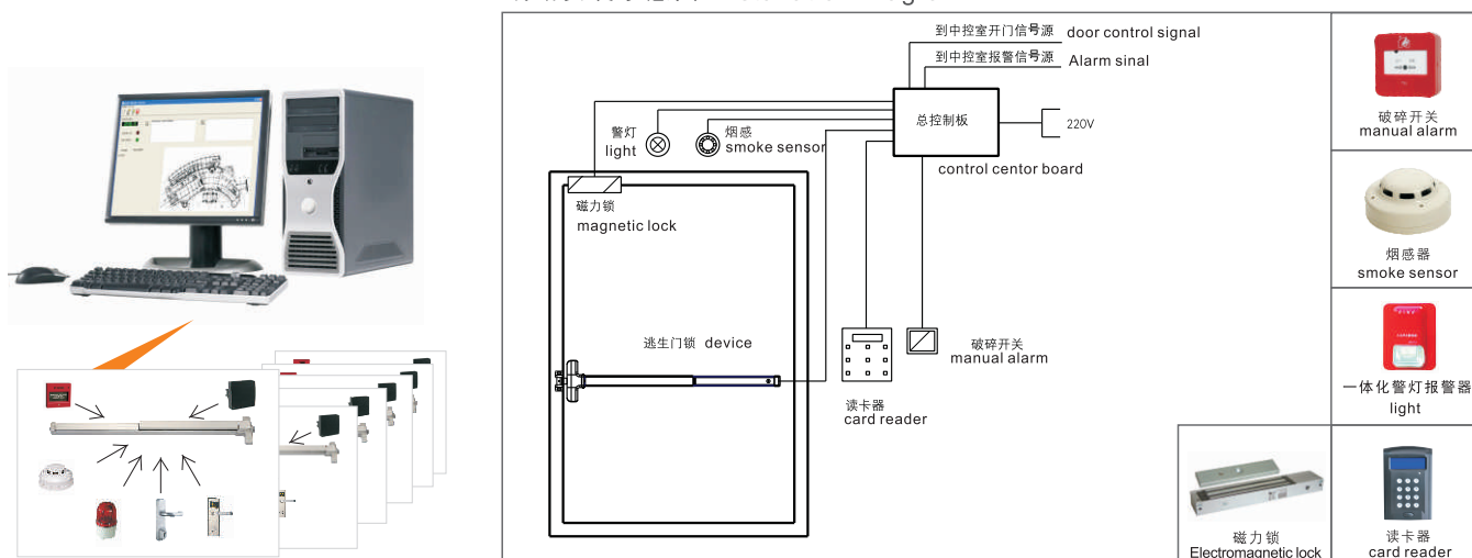
线路安装示意图 Installation Diagram
